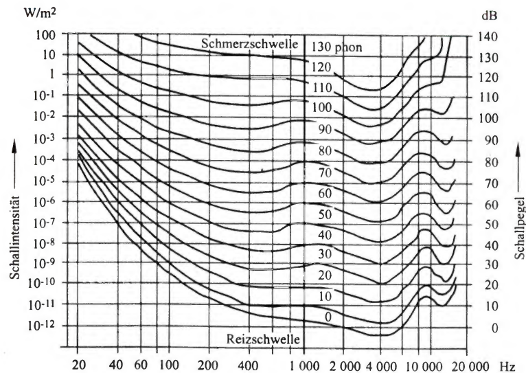
Abbildung 3-1, Kurven gleicher Lautstärke nach Robinson und Dadson
